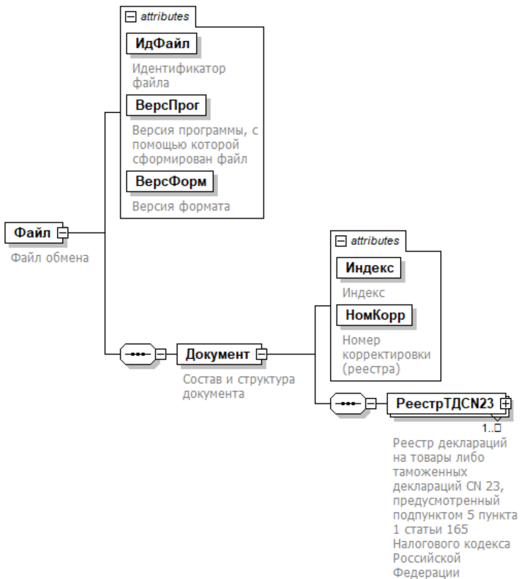
Рисунок 2. Диаграмма структуры файла обмена
