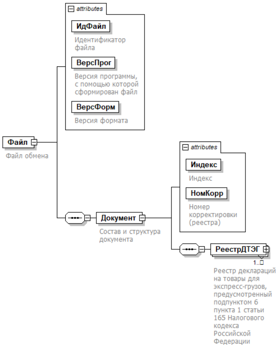
Рисунок 2. Диаграмма структуры файла обмена
