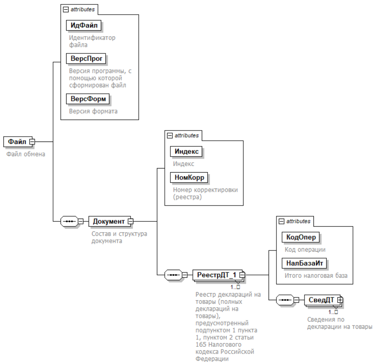
Рисунок 2. Диаграмма структуры файла обмена
